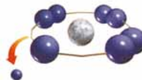
Атом кислорода теряет один электрон: свободный радикал
